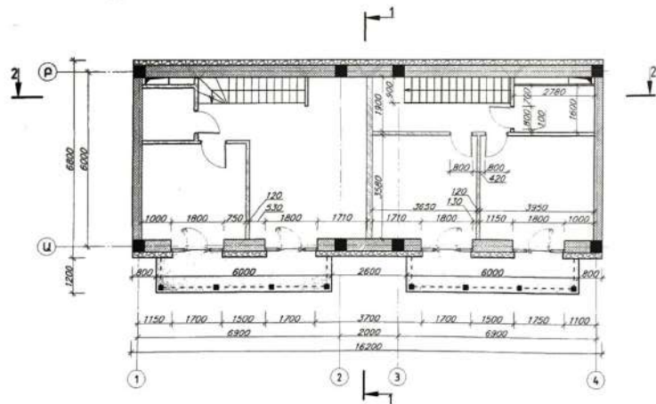
ԵՐԿՐՈՐԴ ՀԱՐԿԻ ՄԻՋՆՈՐՄԵՆԻ ՀԱՏԱԿԱԳԻԾ ՈՍՏ +3.300 ՆԻՇԻ ՀԱՏԱԿԱԳԻԾ Մ 1:100
