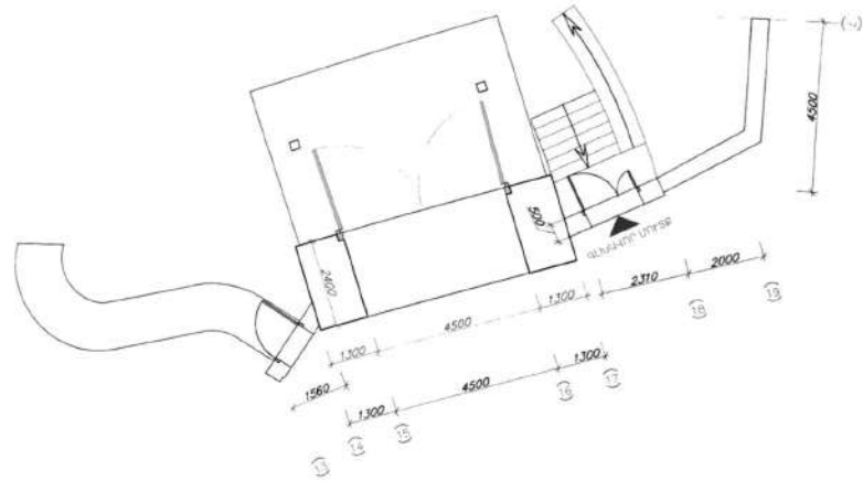
ՊԱՐՄԻԻ ՓՈՎԱԾԸ Մ 1:100
