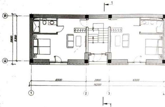
ԱՌԱՋԻՆ ՀԱՐԿԻ ԿԱՀԱՎՈՐՄԱՆ ՀԱՏԱԿԱԳԻԾ Մ 1:100
