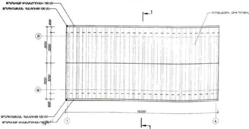
ՏԱՆԻՔԻ ՀԱՏԱԿԱԳԻԾ Մ 1:100
