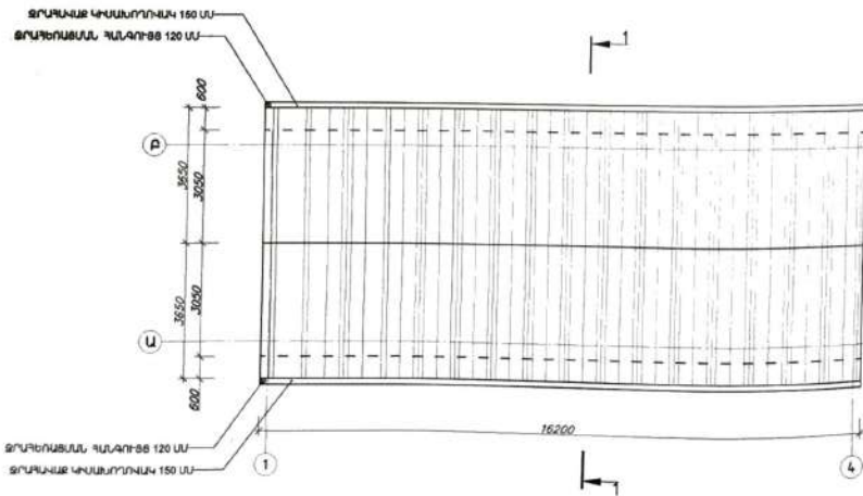
ՏԱՆԻՔԻ ՀԱՏԱԿԱԳԻԾ Մ 1:100
