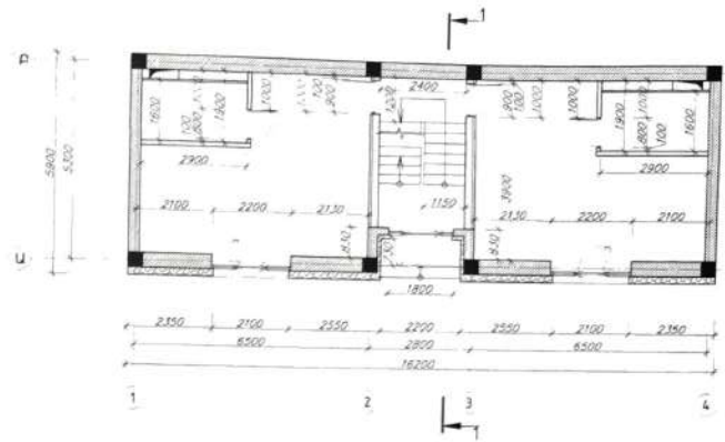
ՄՈՒՋԻՆ ՀԱՐԿԻ ՄԻՋՆՈՐՍԵՐԻ ՀԱՏԱԿԱԳԻԾ ՈՍՏ +0.100 ՆԻՇԻ Մ 1:100
