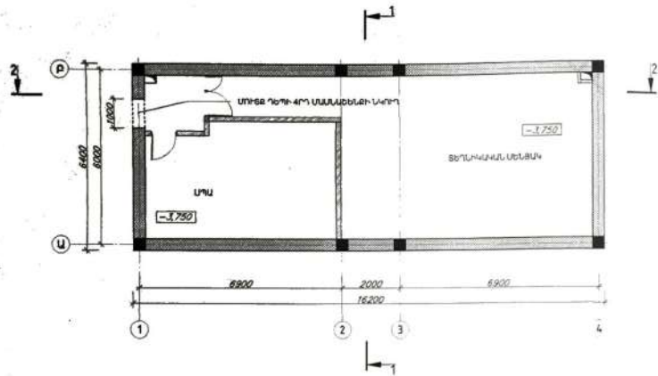
ԵԿՈՒՐԱՅԻՆ ՀԱՐԿԻ ՄԻՋՆՈՐՄԵՆԻ ՀԱՏԱԿԱԳԻԾ ՈՍՏ -3.750 ՆԻՇԻ ՀԱՏԱԿԱԳԻԾ Մ 1:100
