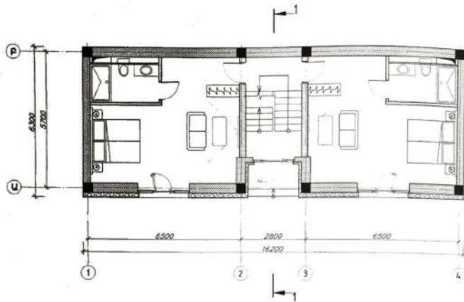
ԱՌՆՔԻՆ ՀԱՐԿԻ ԿԱԿԱԿՈՐՄԱՆ ՀԱՏԱԿԱԳԻԾ Մ 1:100
