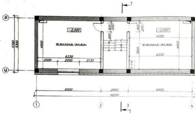
ՆԿՈՒՐԱՅԻՆ ՀԱՐԿԻ ՄԻՋՆՈՐՍԵՐԻ ՀԱՏԱԿԱԳԻԾ ՈՍՏ -2.000 ՆԻՇԻ ՀԱՏԱԿԱԳԻԾ Մ 1:100
