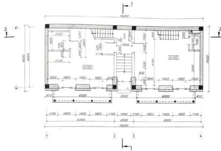
ԱՌԱՋԻՆ ՀԱՐԿԻ ՄԻՋՆՈՐՄԵՆԻ ՀԱՏԱԿԱԳԻԾ ՈՍՏ +0.100 ՆԻՇԻ Մ 1:100
