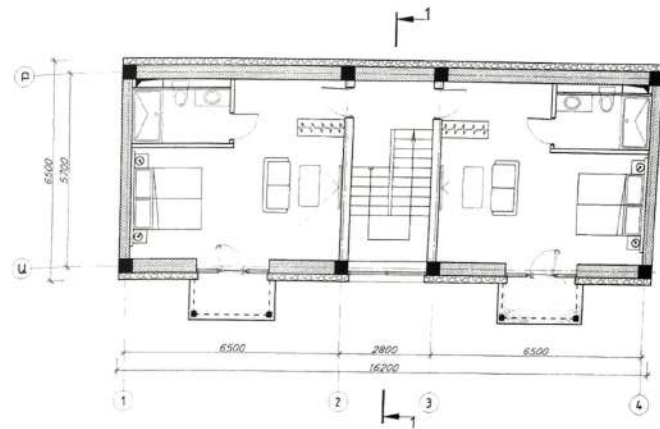
ԵՐԿՐՈՐԴ ՀԱՐԿԻ ԿԱԿԱԿՈՐՄԱՆ ՀԱՏԱԿԱԳԻԾ Մ 1:100
