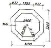
ՇԱՏՐԿԱՆԻ ՀԱՏԱԿԱԳԻԾ Մ 1:100
