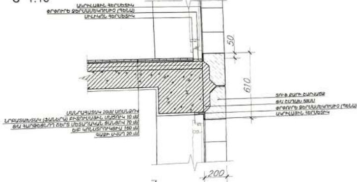
ՏԻՊԱՅԻՆ ՀԱՆՈՒՅՑ Ս 1:15
