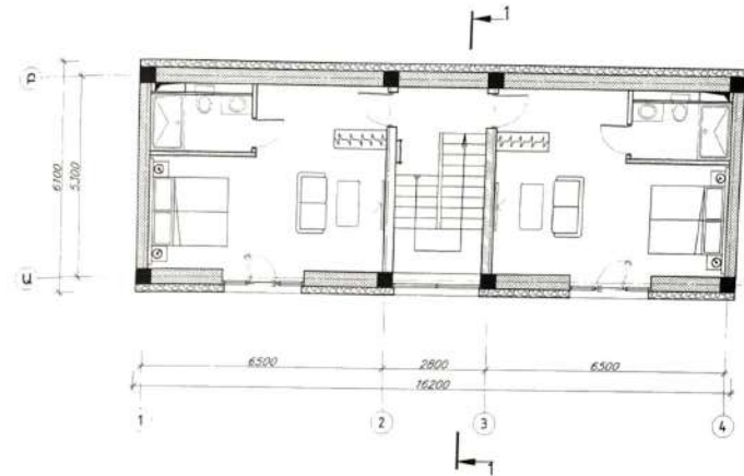
ԵՐԿՐՈՐԴ ՀԱՐԿԻ ԿԱՀԱՎՈՐՄԱՆ ՀԱՏԱԿԱԳԻԾ Մ 1:100
