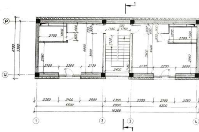
ԵՐԿՐՈՐԴ ՀԱՐԿԻ ՄԻՋՆՈՐՍԵՐԻ ՀԱՏԱԿԱԳԻԾ ՈՍՏ +3.300 ՆԻՇԻ ՀԱՏԱԿԱԳԻԾ Մ 1:100
