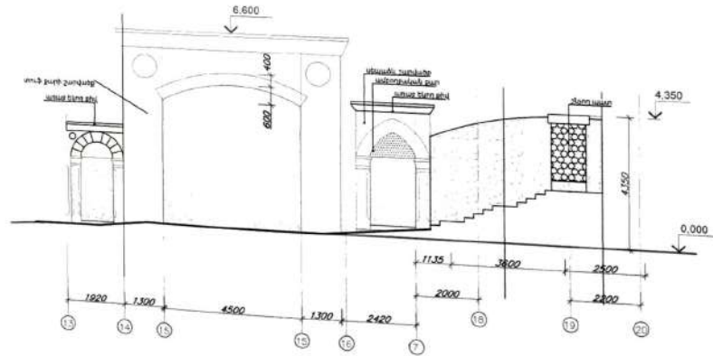
ՊԱՐՄԻԻ ՓՈՎԱԾԸ Մ 1:100
