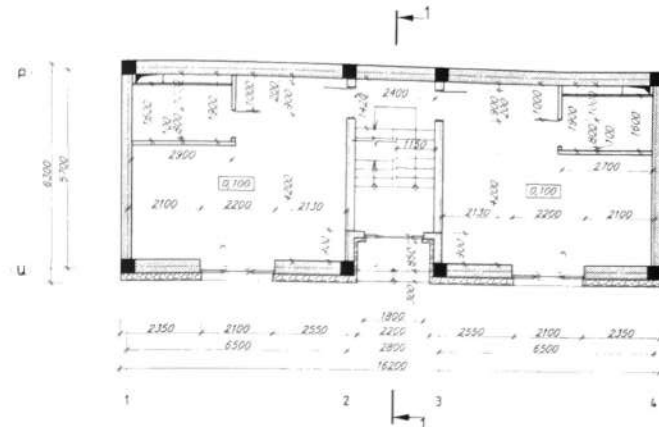
ՄՈՒՋԻՆ ՀԱՐԿԻ ՄԻՋՆՈՐՄԵՐԻ ՀԱՏԱԿԱԳԻԾ ՈՒՏ +0.100 ՆԻՇԻ Մ 1:100
