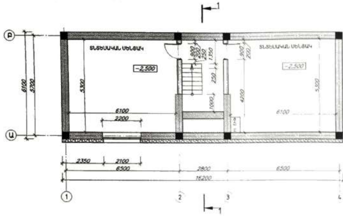
ՆԿՈՒԱՅԻՆ ՀԱՐԿԻ ՄԻՋՆՈՐՄԵՐԻ ՀԱՏԱԿԱԳԻԾ ՈՒՏ -2.500 ՆԻՇԻ ՀԱՏԱԿԱԳԻԾ Մ 1:100
