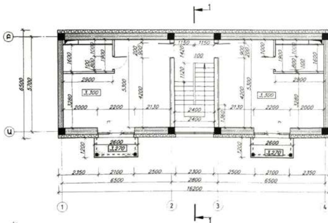
ԵՐԿՐՈՐԴ ՀԱՐԿԻ ՄԻՋՆՈՐՄԵՐԻ ՀԱՏԱԿԱԳԻԾ ՈՒՏ +3.300 ՆԻՇԻ ՀԱՏԱԿԱԳԻԾ Մ 1:100
